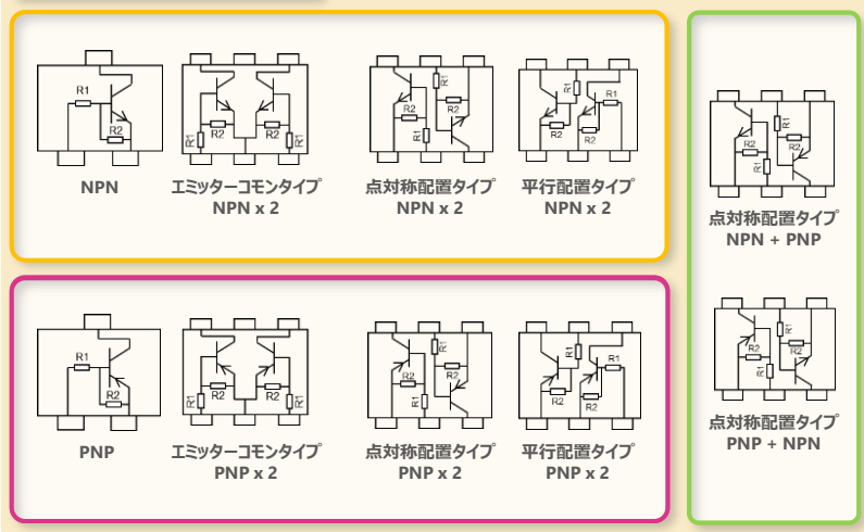
内部接続図
