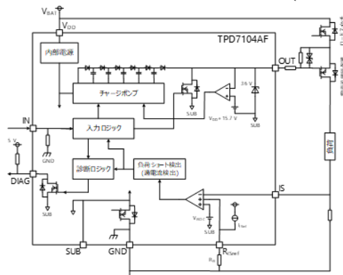
バック・トゥ・バック構成
