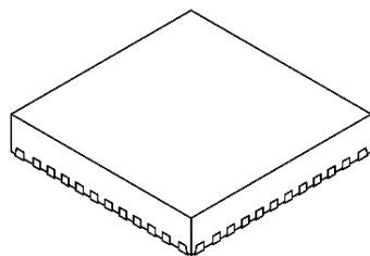
パッケージ: P-WQFN40-0606-0.50-001 (6 x 6 x 0.8 mm)
