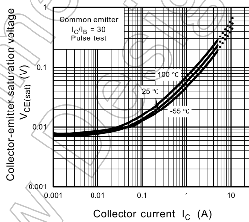
Fig. 7.4 V_{CE(sat)} - I_C
