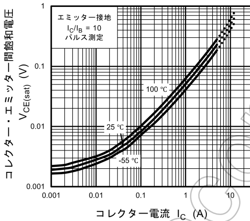
図 7.3 V_{CE(sat)} - I_C
