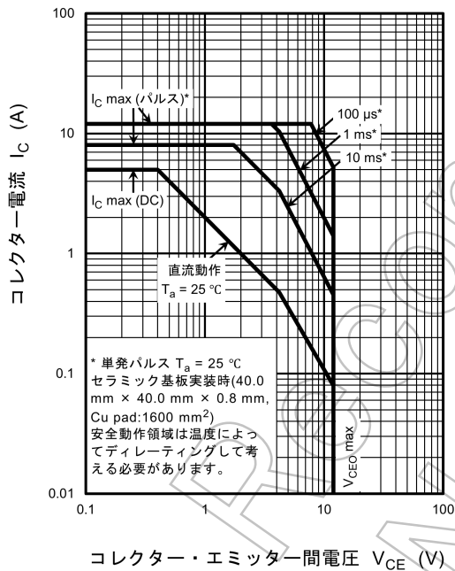
図 7.8 安全動作領域 (最大値 (保証値))
