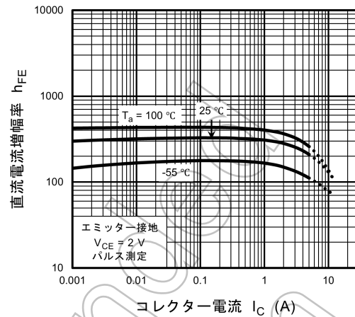
図 7.2 h_{FE} - I_C
