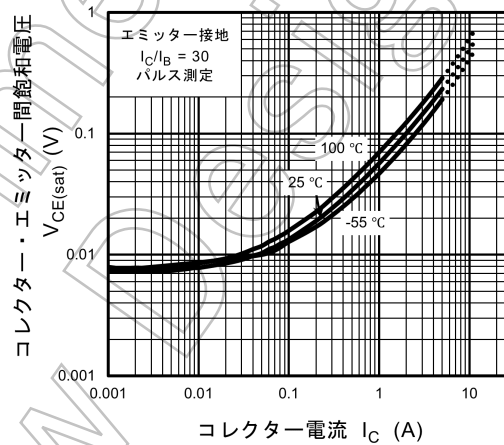
図 7.4 V_{CE(sat)} - I_C
