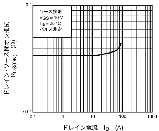
図 8.6 R_{DS(ON)} - I_D
