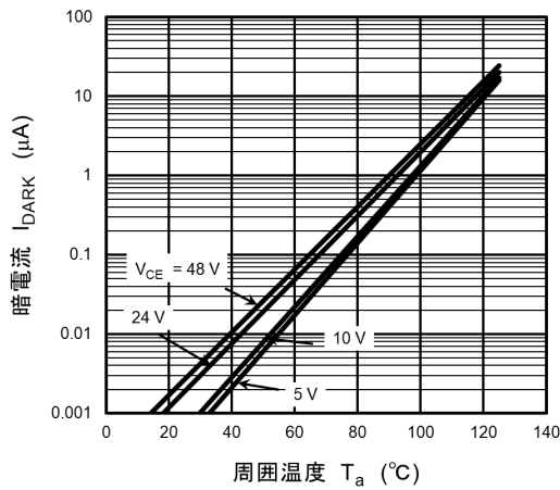
図 12.9 I_{DARK} - T_a
