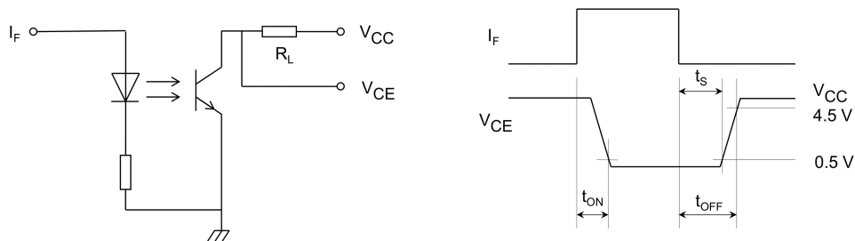
図 11.1 スイッチング時間測定回路, 波形
