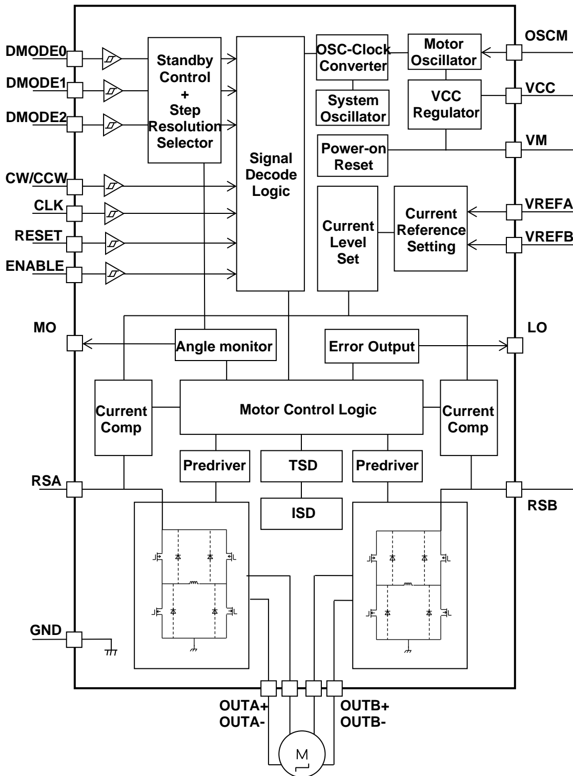
図 3.1 ブロック図
