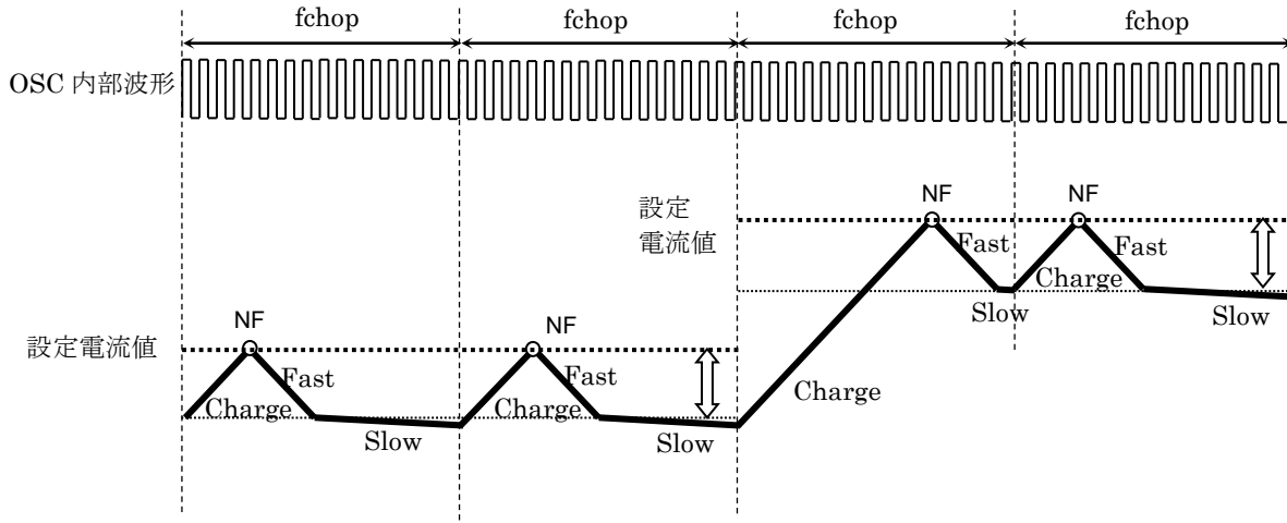
図 6.11 設定電流値が増加方向の場合
