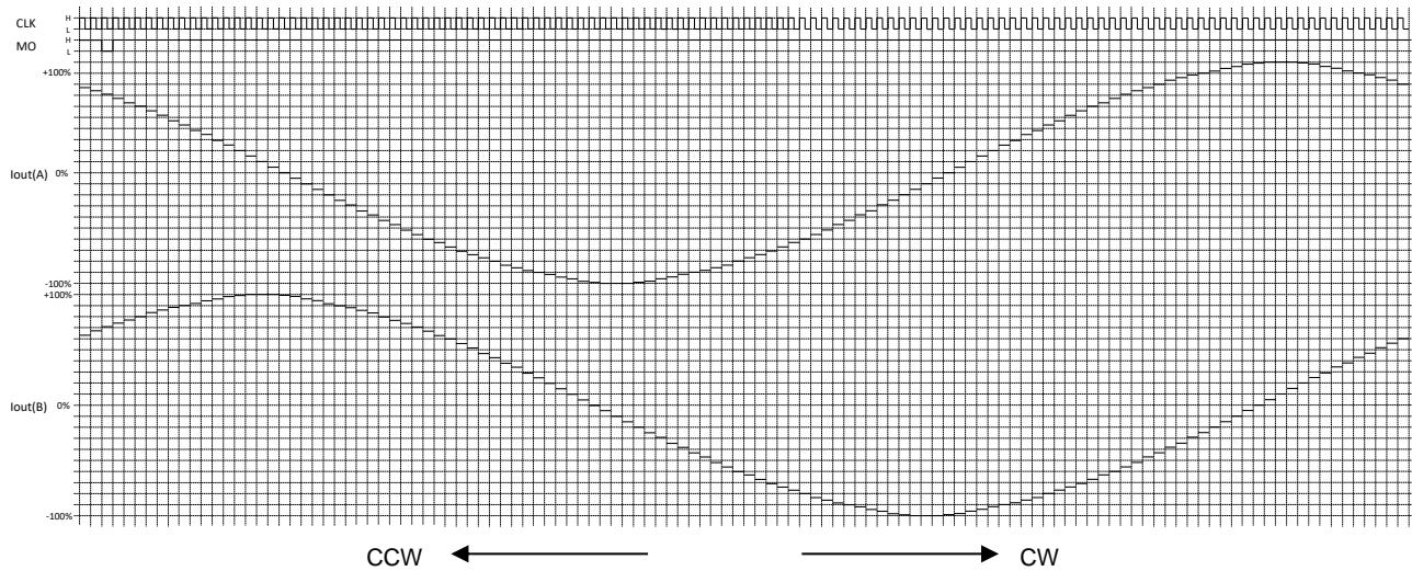
図 6.7 8W1-2 相励磁設定
