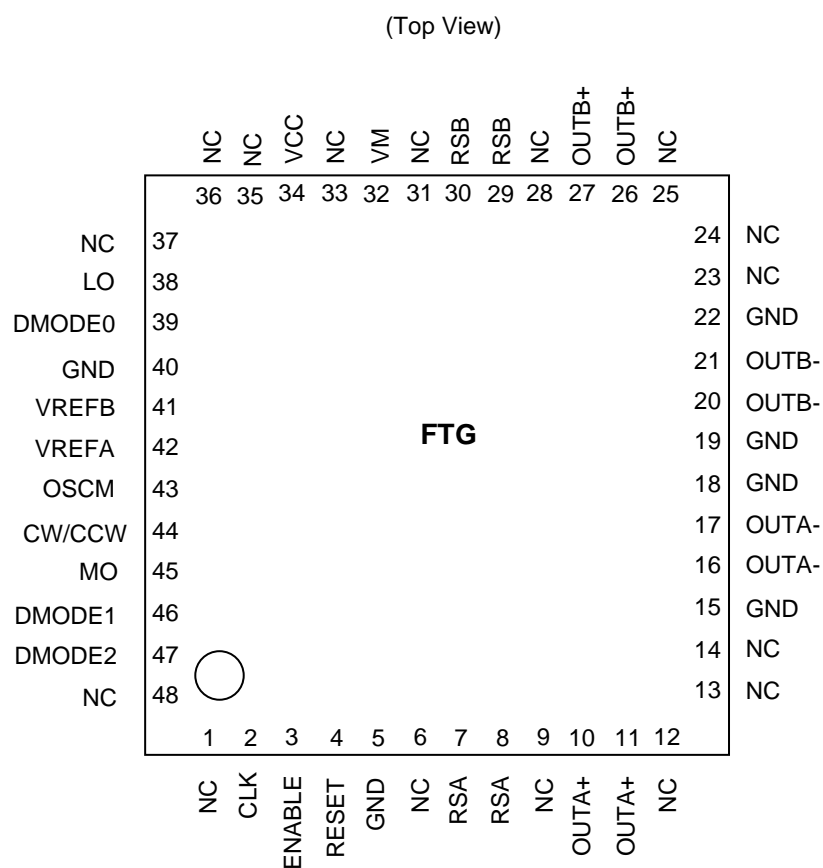
図 4.1 端子配置図
