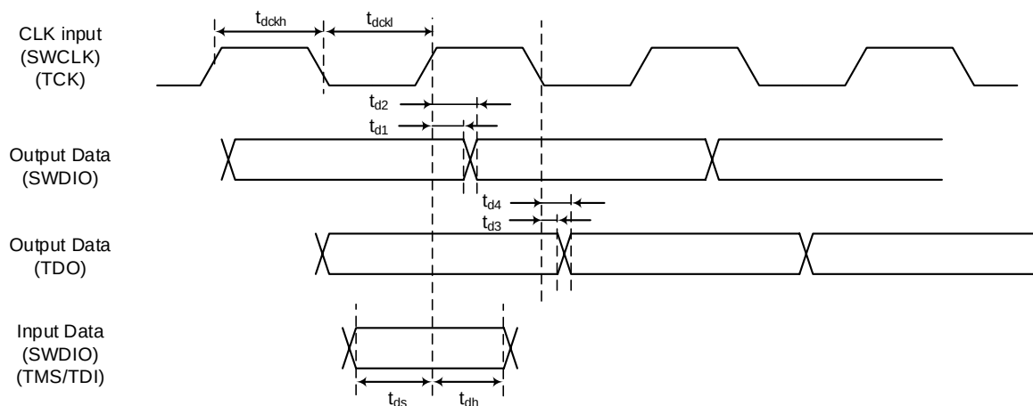
図 7.10 JTAG/SW波形
