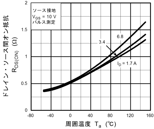
図 8.7 R_{DS(ON)} - T_a
