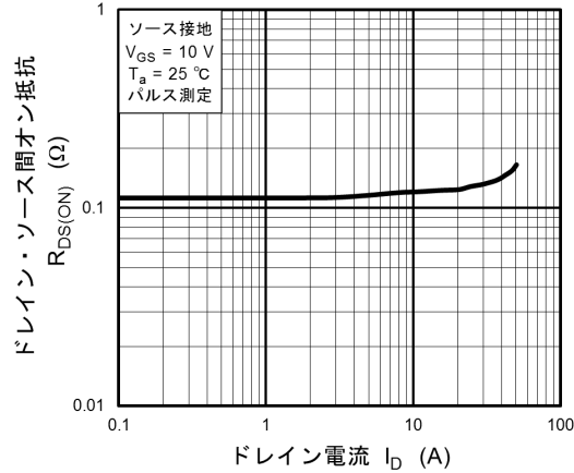
図 8.6 R_{DS(ON)} - I_D
