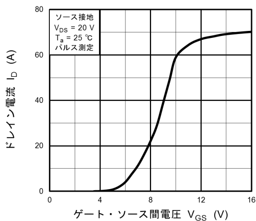
図 8.3 I_D - V_{GS}
