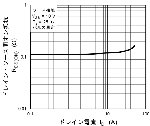
図 8.6 R_{DS(ON)} - I_D
