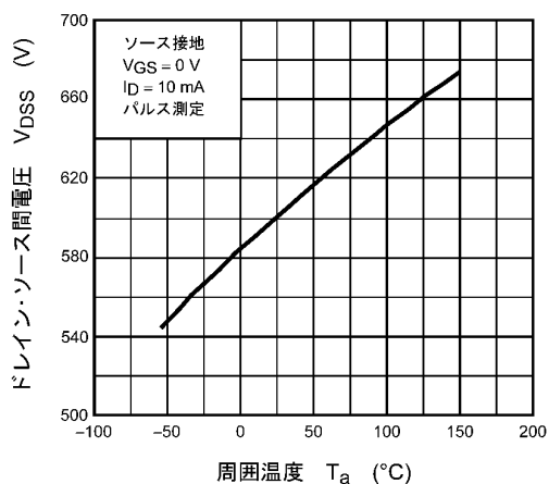
図 8.5 V_{DS} - T_a
