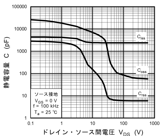
図 8.9 C - V_{DS}
