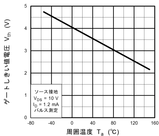
図 8.11 V_{th} - T_a
