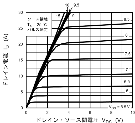
図 8.1 I_D - V_{DS}
