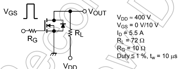
図 6.2.1 スwitching時間の測定回路例
