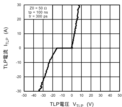
図 10.13.1 I_{TLP} - V_{TLP}
