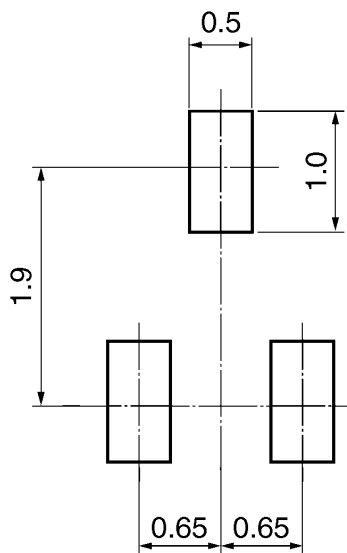
図 9.1 参考パッド寸法(Unit: mm)
