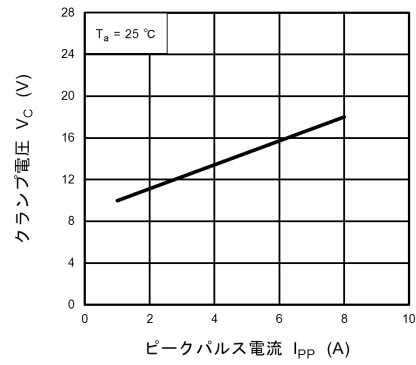
図 10.7.2 V_C - I_{PP}
