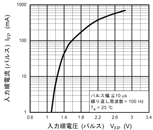
図 11.6 I_{FP} - V_{FP}
