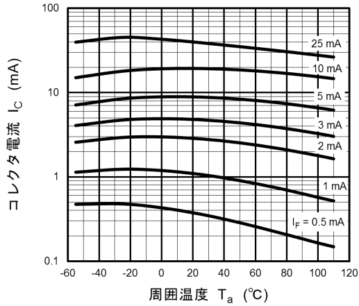
図 11.13 I_C - T_a
