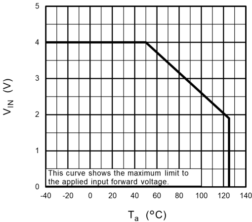
Fig. 12.1 V_{IN} - T_a
