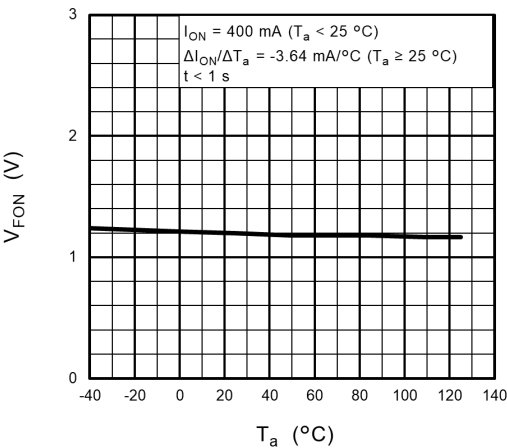
Fig. 12.6 V_{FON} - T_a
