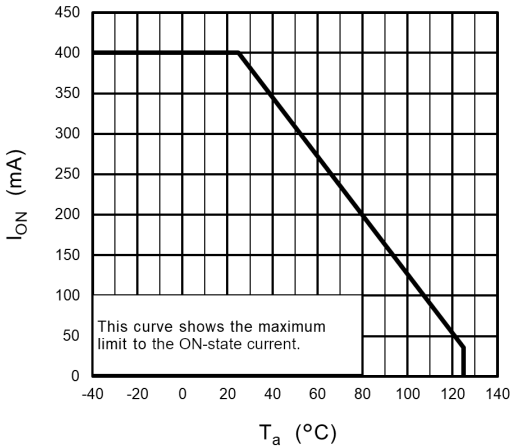
Fig. 12.3 I_{ON} - T_a
