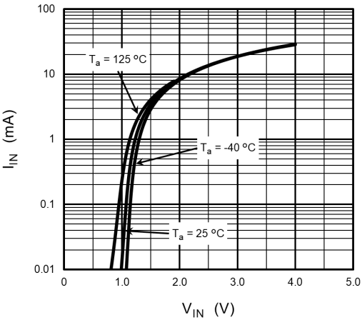
Fig. 12.2 I_{IN} - V_{IN}
