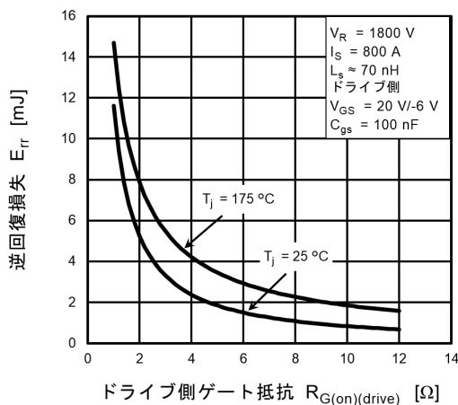
図 9.3 E_{rr} - R_{G(on)}
