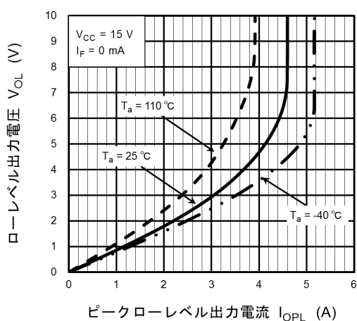
図 13.2.9 V_{OL} - I_{OPL}
