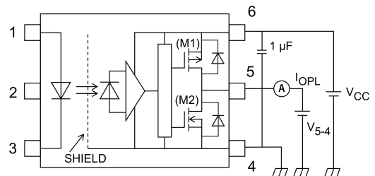
図 13.1.2 I_{OPL} 測定回路
