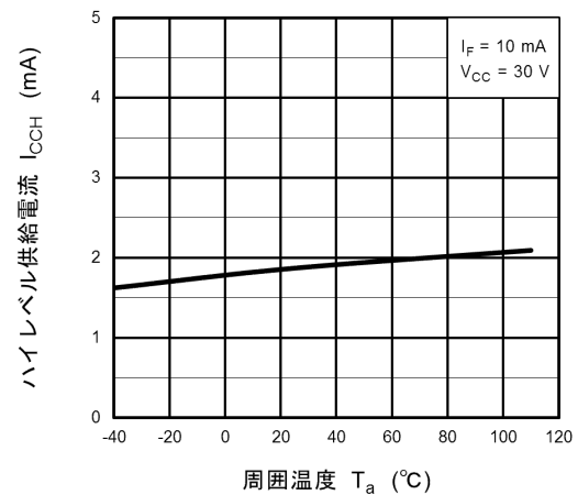
図 13.2.6 I_{CCH} - T_a
