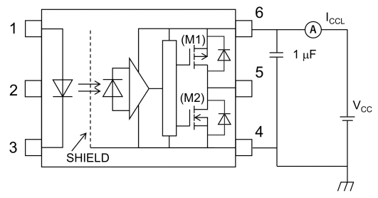
図 13.1.6 I_{CCL} 測定回路
