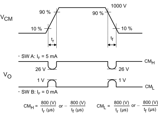
図 13.1.8 コモンモード過渡耐性測定回路, 波形
