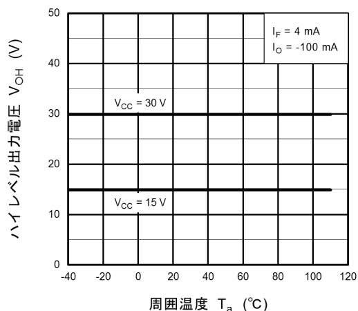
図 13.2.8 V_{OH} - T_a
