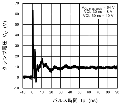
図 10.5.5 ISO10605 クランプ波形 +8 kV
