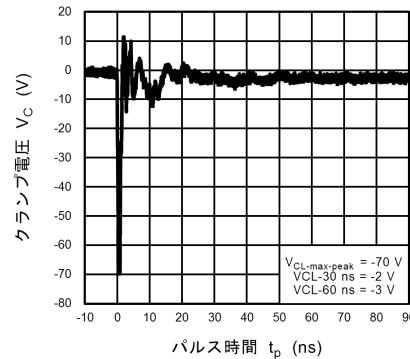
図 10.13.6 ISO10605 クランプ波形 -8 kV
