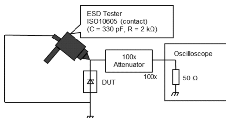
図 10.22.3 クランプ波形測定回路 (ISO10605準拠)
