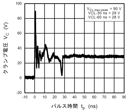
図 10.17.5 ISO10605 クランプ波形 +8 kV
