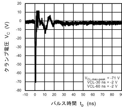
図 10.14.6 ISO10605 クランプ波形 -8 kV
