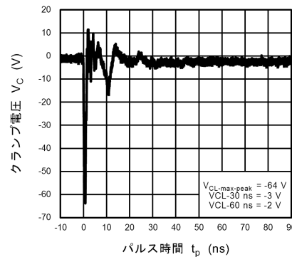
図 10.16.6 ISO10605 クランプ波形 -8 kV
