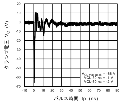
図 10.2.6 ISO10605 クランプ波形 -8 kV
