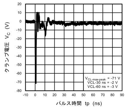
図 10.4.6 ISO10605 クランプ波形 -8 kV
