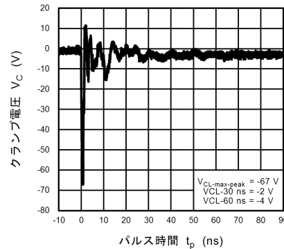
図 10.15.6 ISO10605 クランプ波形 -8 kV
