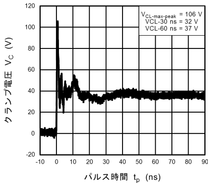
図 10.19.5 ISO10605 クランプ波形 +8 kV
