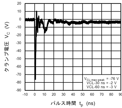
図 10.10.6 ISO10605 クランプ波形 -8 kV
