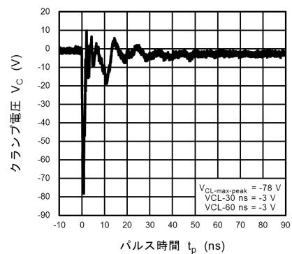
図 10.21.6 ISO10605 クランプ波形 -8 kV
