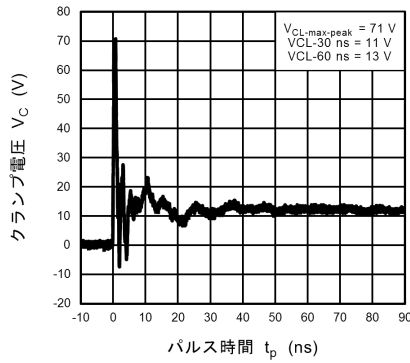
図 10.8.5 ISO10605 クランプ波形 +8 kV
