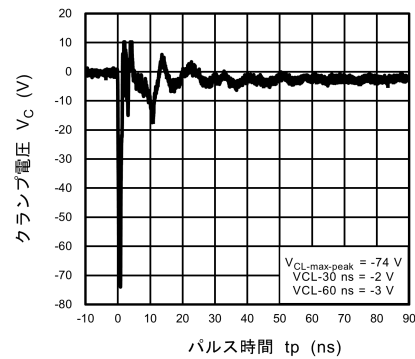
図 10.6.6 ISO10605 クランプ波形 -8 kV
