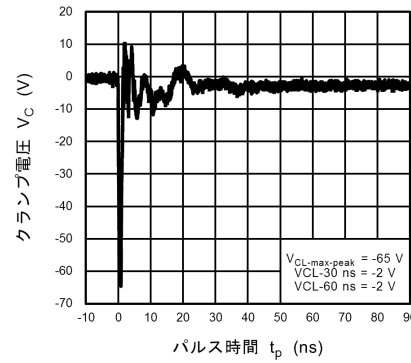
図 10.8.6 ISO10605 クランプ波形 -8 kV
