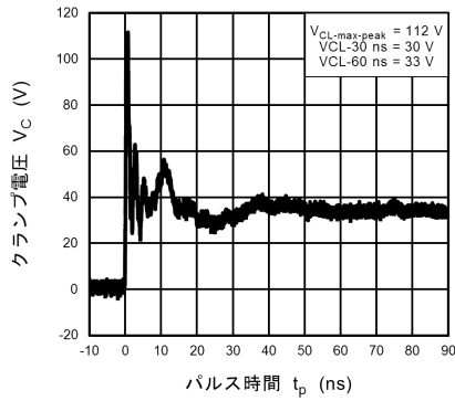
図 10.18.5 ISO10605 クランプ波形 +8 kV
