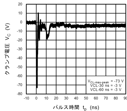
図 10.11.6 ISO10605 クランプ波形 -8 kV
