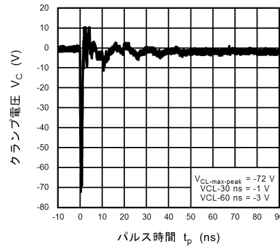
図 10.12.6 ISO10605 クランプ波形 -8 kV
