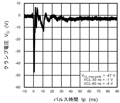
図 10.5.6 ISO10605 クランプ波形 -8 kV
