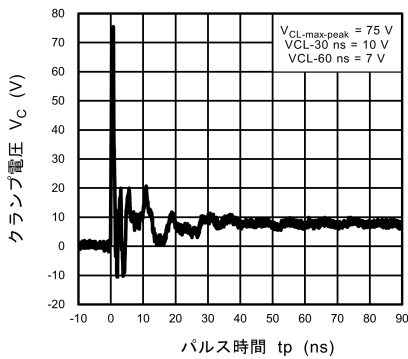
図 10.3.5 ISO10605 クランプ波形 +8 kV
