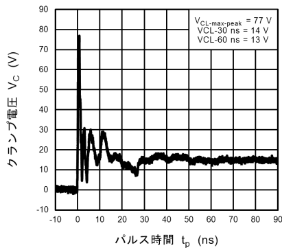
図 10.9.5 ISO10605 クランプ波形 +8 kV
