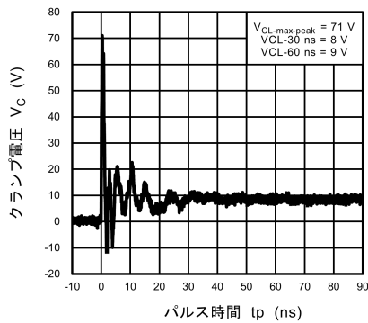
図 10.4.5 ISO10605 クランプ波形 +8 kV
