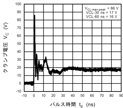
図 10.11.5 ISO10605 クランプ波形 +8 kV
