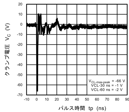
図 10.3.6 ISO10605 クランプ波形 -8 kV
