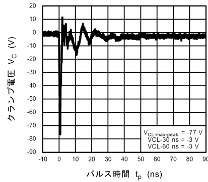
図 10.18.6 ISO10605 クランプ波形 -8 kV
