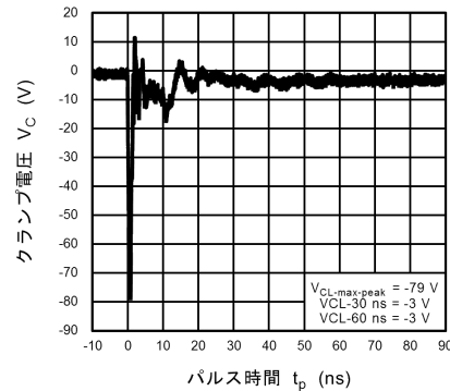
図 10.19.6 ISO10605 クランプ波形 -8 kV
