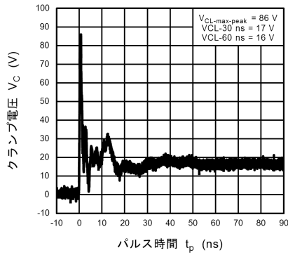
図 10.10.5 ISO10605 クランプ波形 +8 kV
