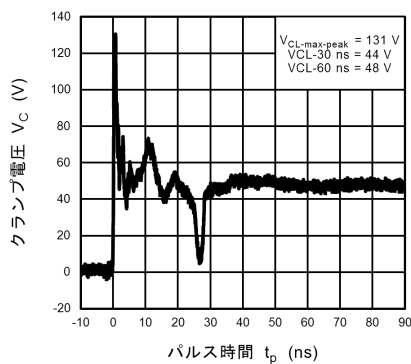
図 10.21.5 ISO10605 クランプ波形 +8 kV
