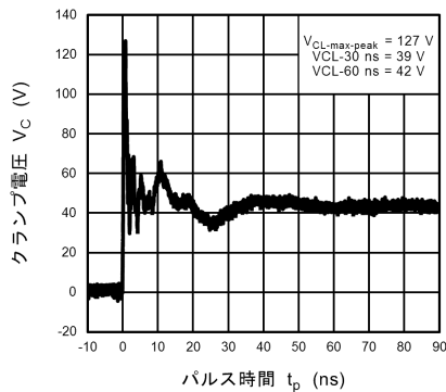
図 10.20.5 ISO10605 クランプ波形 +8 kV
