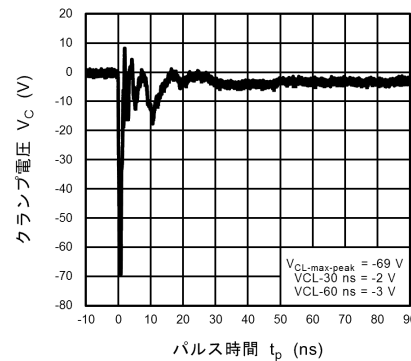
図 10.9.6 ISO10605 クランプ波形 -8 kV
