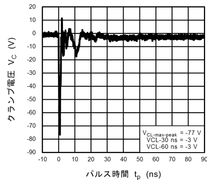
図 10.20.6 ISO10605 クランプ波形 -8 kV
