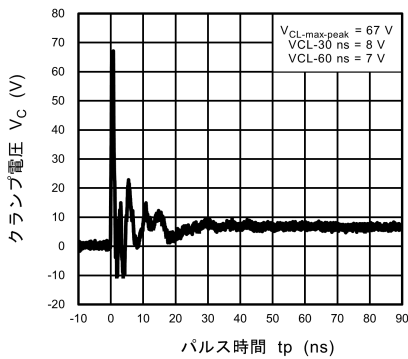
図 10.2.5 ISO10605 クランプ波形 +8 kV
