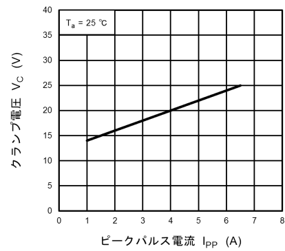
図 10.11.2 V_C - I_{pp}
