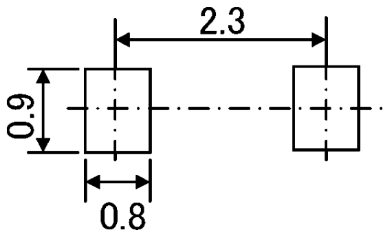
図 9.1 参考パッド寸法(Unit: mm)
