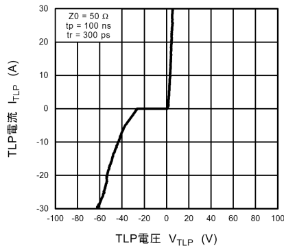
図 10.18.1 I_{TLP} - V_{TLP}
