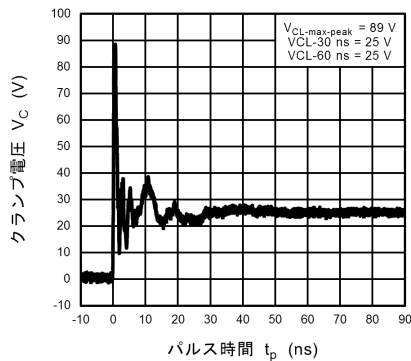
図 10.16.5 ISO10605 クランプ波形 +8 kV
