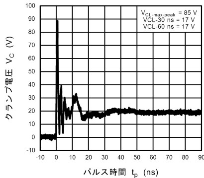
図 10.13.5 ISO10605 クランプ波形 +8 kV
