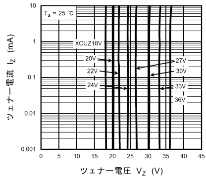
図 10.1.2 I_Z - V_Z(2)
