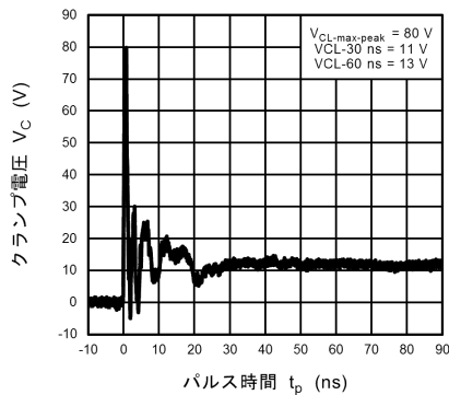
図 10.7.5 ISO10605 クランプ波形 +8 kV
