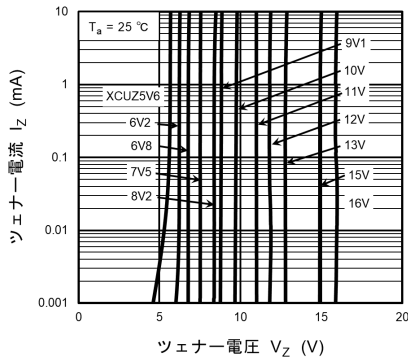
図 10.1.1 I_Z - V_Z(1)
