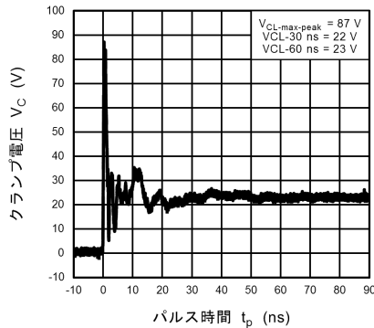
図 10.15.5 ISO10605 クランプ波形 +8 kV
