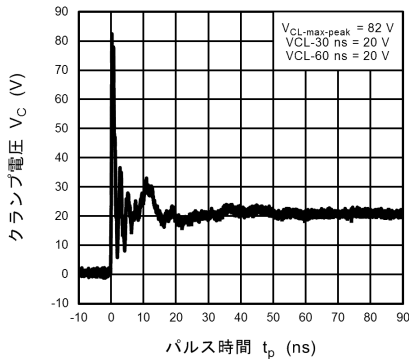
図 10.14.5 ISO10605 クランプ波形 +8 kV
