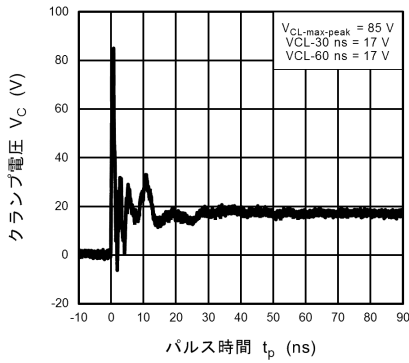
図 10.12.5 ISO10605 クランプ波形 +8 kV
