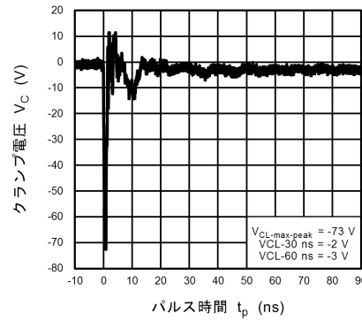
図 10.17.6 ISO10605 クランプ波形 -8 kV
