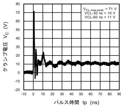
図 10.6.5 ISO10605 クランプ波形 +8 kV
