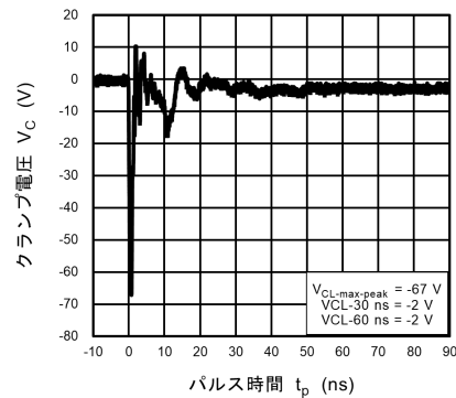
図 10.7.6 ISO10605 クランプ波形 -8 kV
