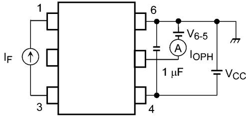
图 13.1.1 IOPH测定回路
