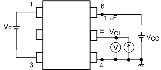
图 13.1.4 VOL测定回路
