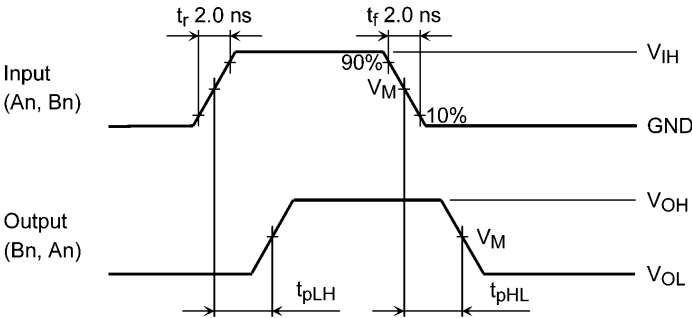
図 13.1 tPLH, tPHL
