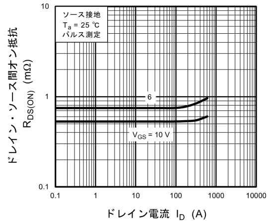
図 8.8 R_{DS(ON)} - I_D
