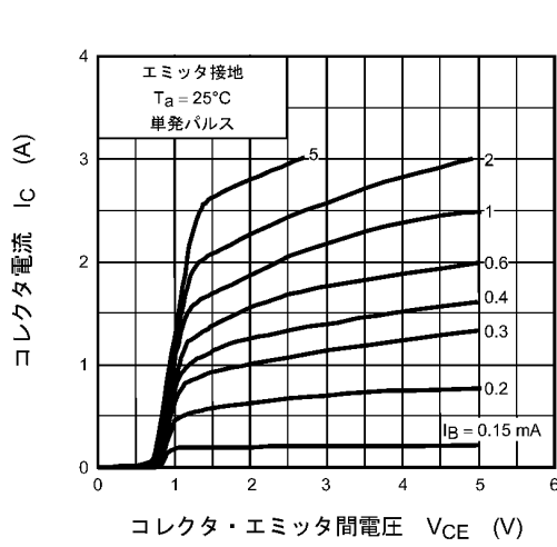
図 8.1.1 IC - VCE
