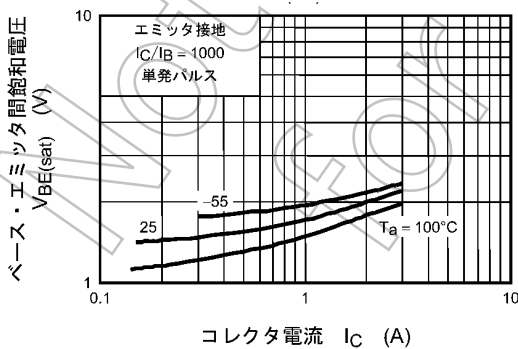
図 8.1.5 VBE(sat) - IC
