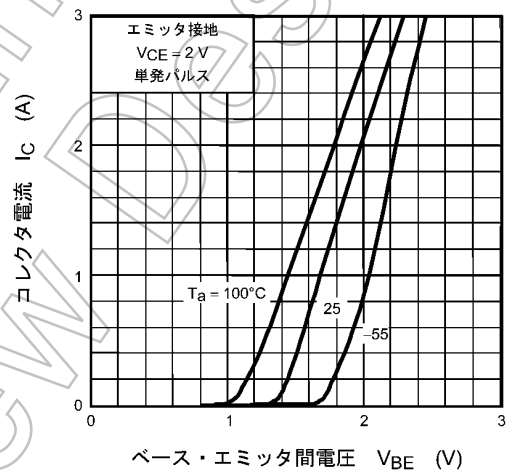
図 8.1.4 IC - VBE
