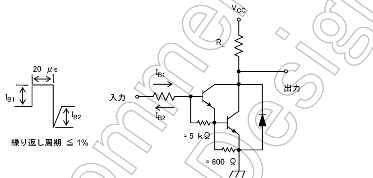
図 5.1.1 スwitching時間測定回路
