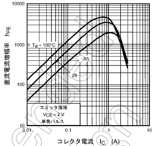
図 8.1.2 hFE - IC
