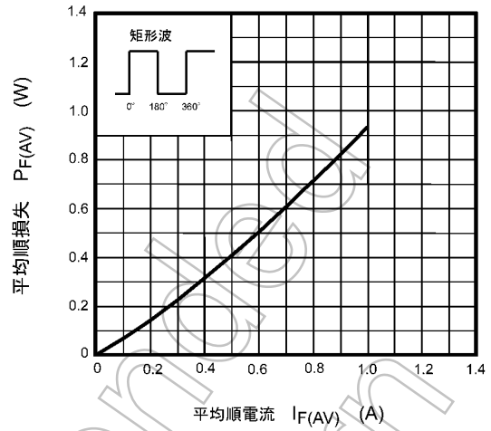
図 8.2.2 P_{F(AV)} - I_{F(AV)}
