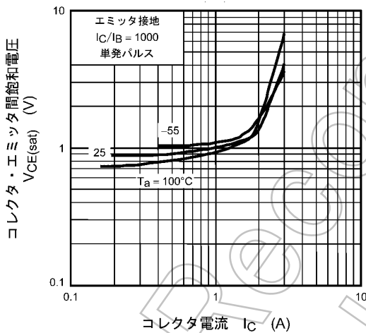
図 8.1.3 VCE(sat) - IC
