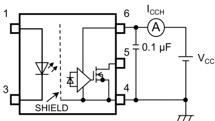
図 12.1.3 I CCH 測定回路
