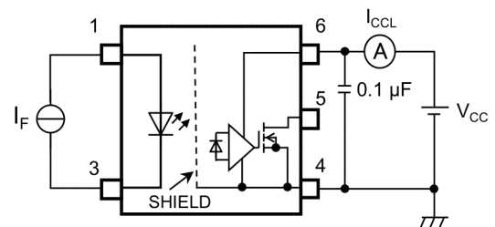
図 12.1.4 I CCL 測定回路
