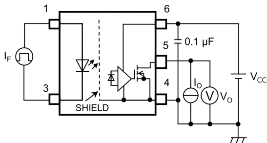
図 12.1.5 I FHL , I FLH , I HYS 測定回路
