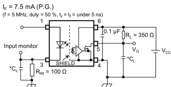
Fig. 12.1.5 I_{FHL} , I_{FLH} , I_{HYS} Test Circuit
