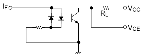
図 2: スwitchング時間測定回路
