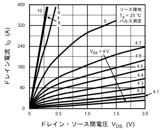
図 8.2 I_D - V_{DS}
