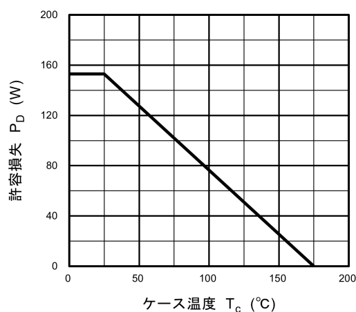
図 8.16 P_D - T_c (最大値 (保証値))
