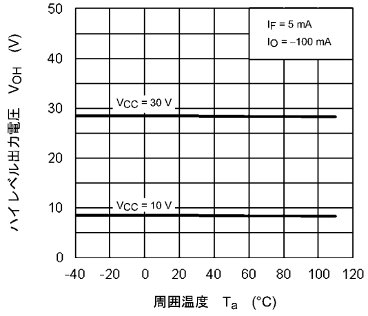
図 13.2.8 V_{OH} - T_a
