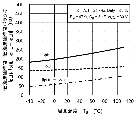
図 13.2.11 t_{pLH}, t_{pHL}, |t_{pHL} - t_{pLH}| - T_a
