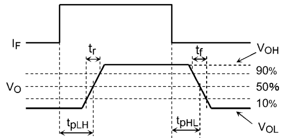
图 13.1.7 伝搬遅延時間測定回路, 波形
