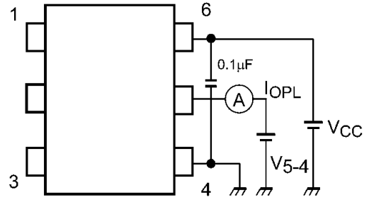
图 13.1.2 I OPL 测定回路
