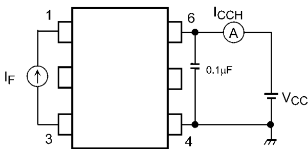
图 13.1.5 I CCH 测定回路
