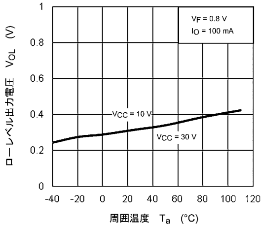
図 13.2.7 V_{OL} - T_a
