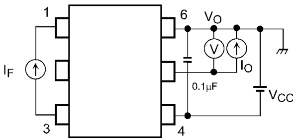
图 13.1.1 I OPH 测定回路
