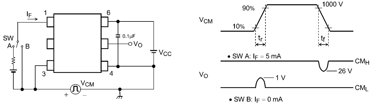
图 13.1.8 コモンモード過渡耐性測定回路, 波形
