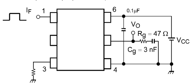
图 13.1.7 伝搬遅延時間測定回路, 波形
