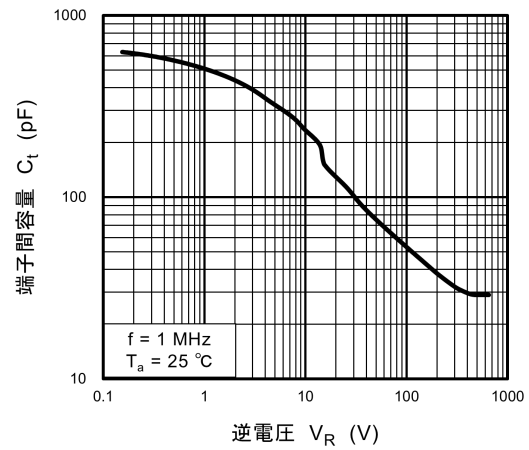
図 9.4 C_t - V_R
