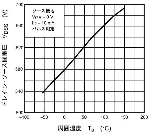
図 8.5 V_{DSS} - T_a
