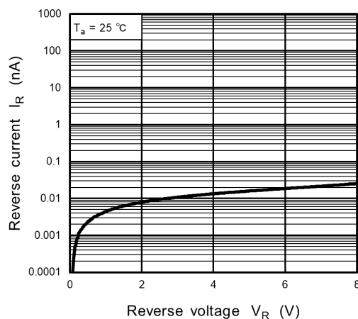
図 7.2 I_R - V_R
