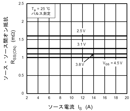
図 9.2 R_{SS(ON)} - I_S
