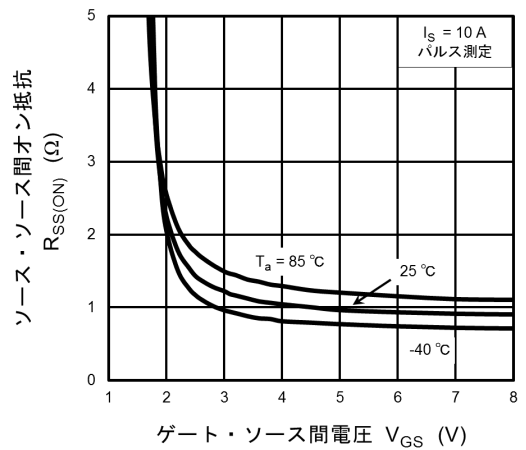
図 9.4 R_{SS(ON)} - V_{GS}
