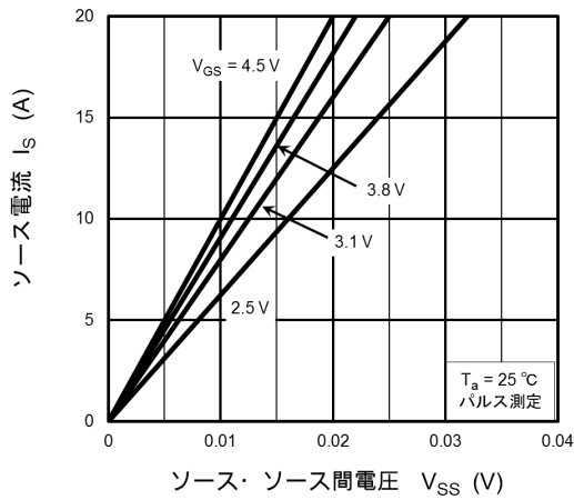
図 9.1 I_S - V_{SS}
