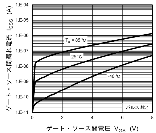
図 9.6 I_{GSS} - V_{GS}
