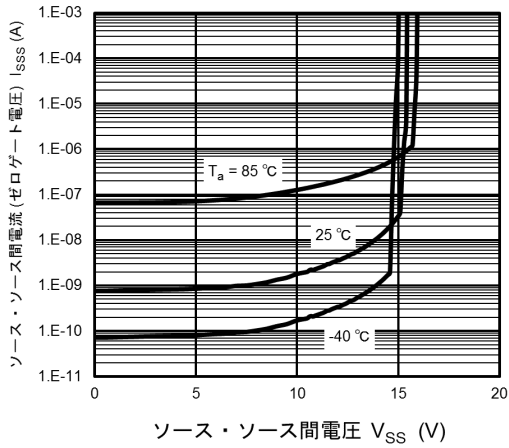
図 9.7 I_{SSS} - V_{SS}
