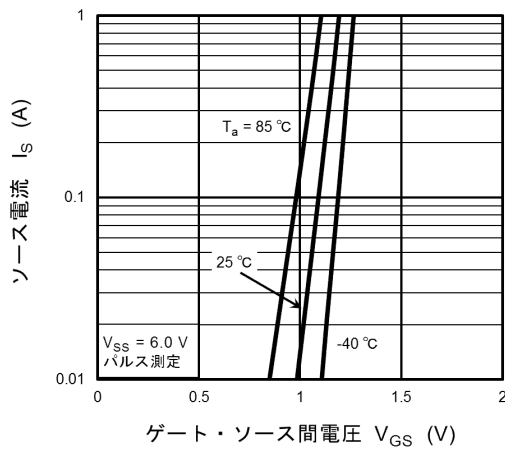
図 9.3 I_S - V_{GS}
