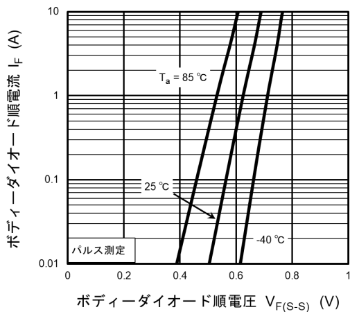
図 9.5 I_F - V_{F(S-S)}
