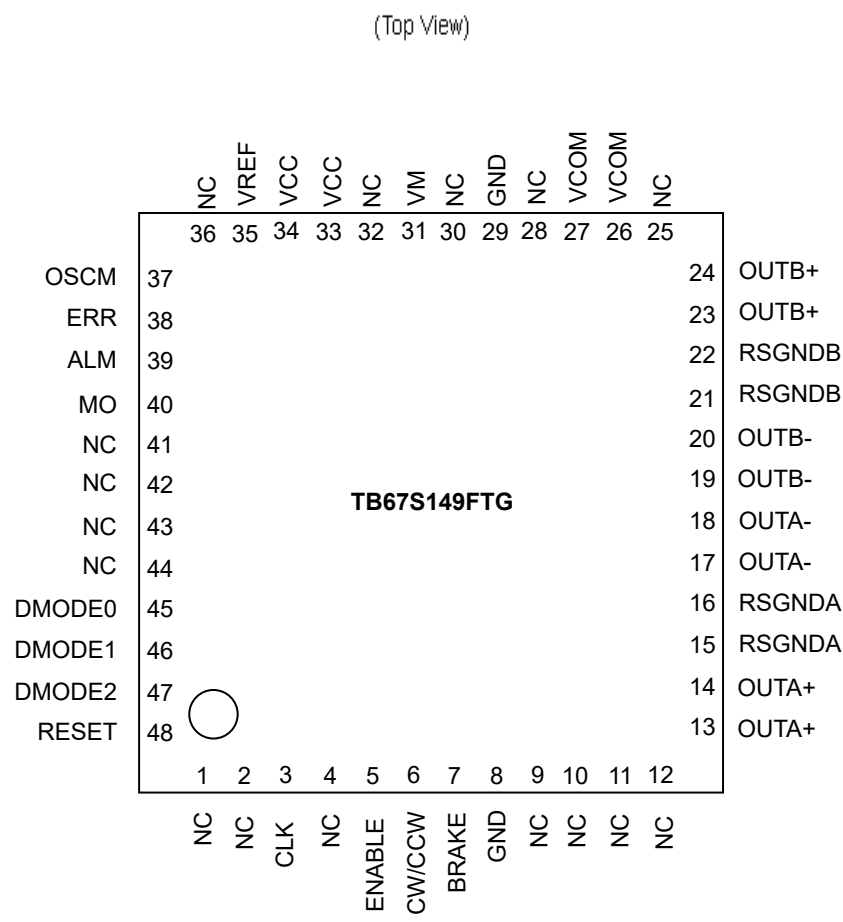
図 4.1 端子配置図
