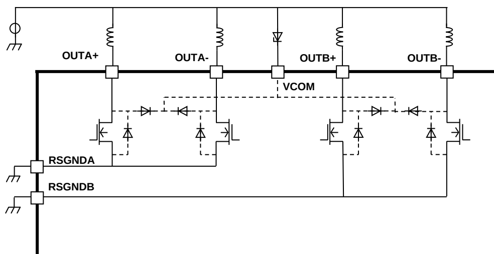
図 6.1 BRAKE モード等価回路
