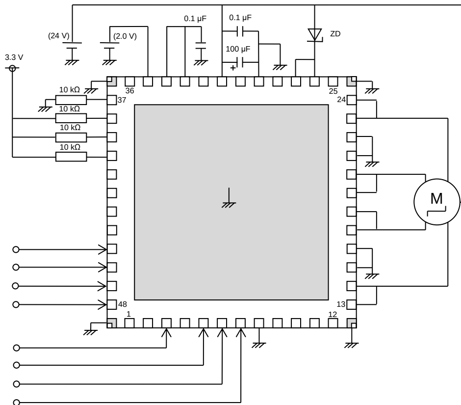
図 10.1 応用回路例
