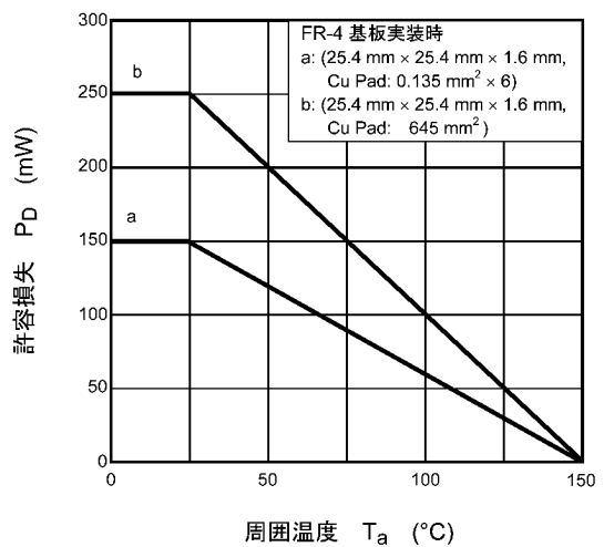
図 7.12 P_D - T_a
