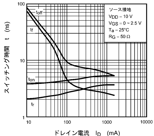
図 7.10 t - I_D
