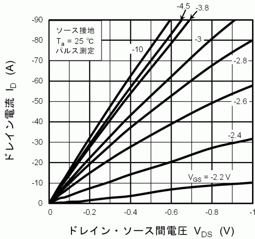
図 8.1 I_D - V_{DS}
