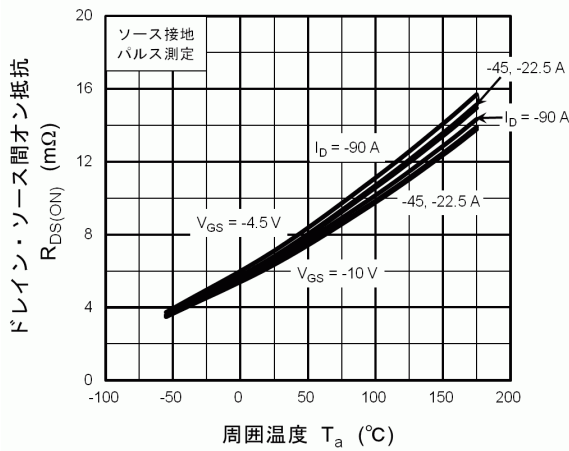
図 8.9 R_{DS(ON)} - T_a
