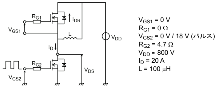
図 6.2.1 スwitchング時間の測定回路
