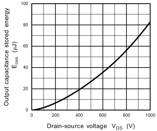
Fig. 8.14 E oss - V DS
