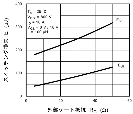
図 8.16 E - R_G
