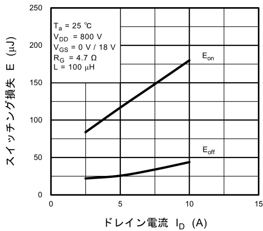
図 8.15 E - I_D
