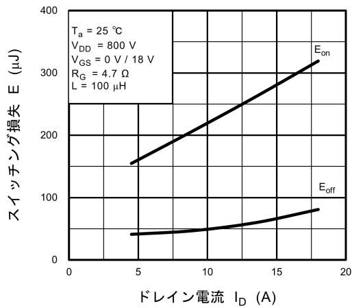
図 8.15 E - I_D
