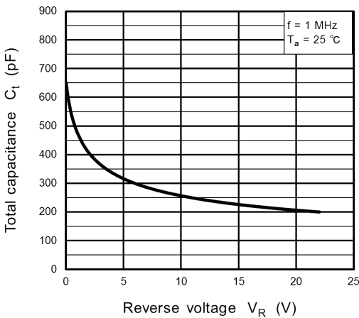
図 9.3 C_t - V_R
