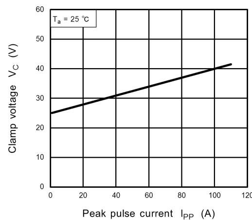
図 6.3.1 V_C - I_{PP}
