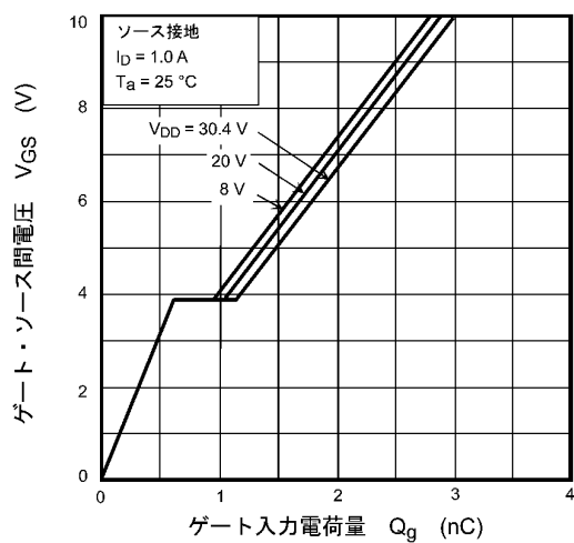
図 7.11 ダイナミック入力特性
