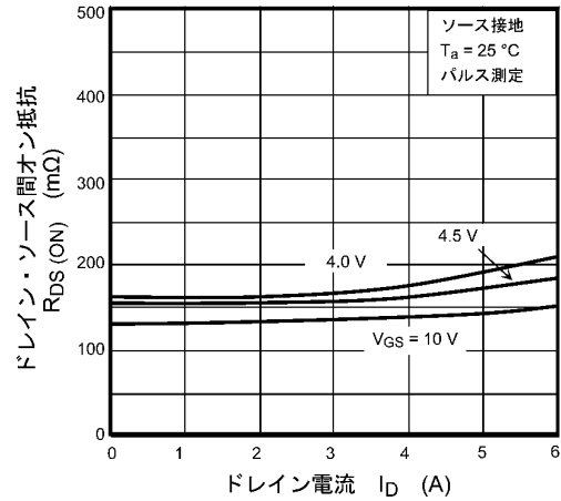
図 8.4 R_{DS(ON)} - I_D
