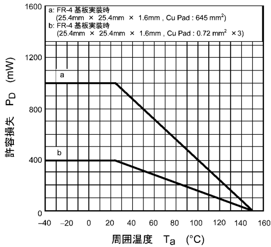
図 7.15 P_D - T_a
