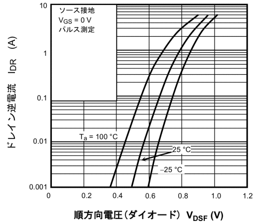
図 8.8 I_{DR} - V_{DSF}
