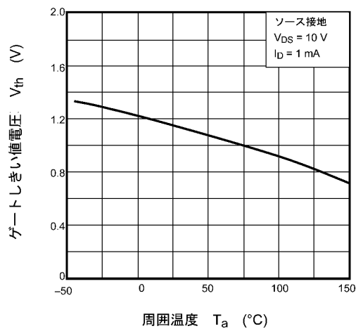
図 7.6 V_{th} - T_a
