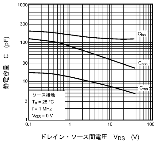
図 7.9 C - V_{DS}
