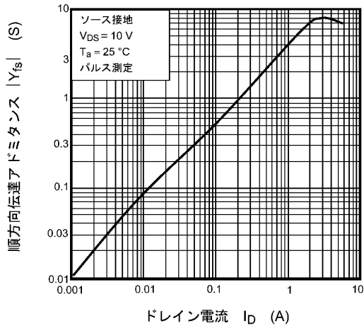
図 7.7 |Y_{fs}| - I_D
