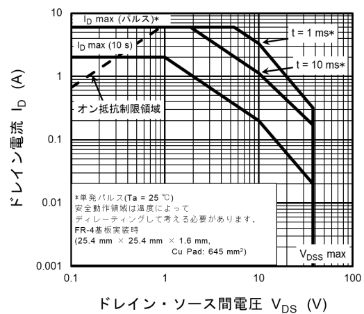
図 7.12 安全動作領域
