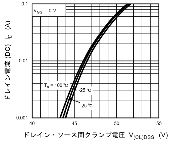
図 7.14 I_D - V_{(CL)DSS}
