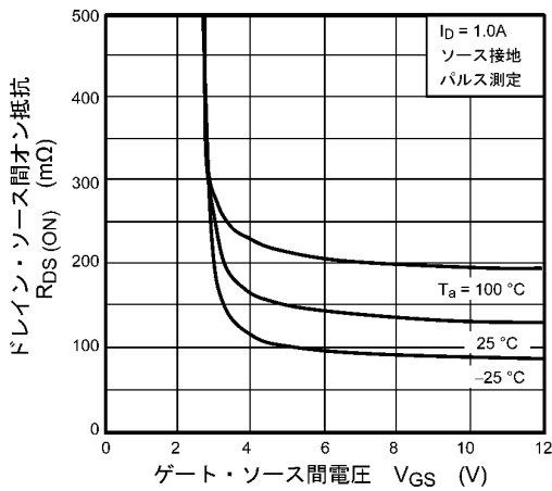
図 8.3 R_{DS(ON)} - V_{GS}
