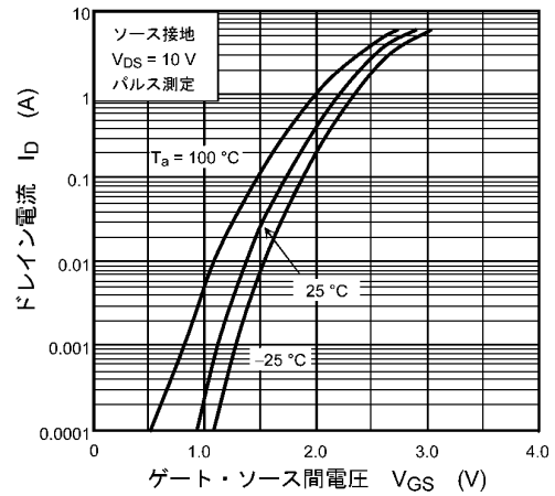
図 8.2 I_D - V_{GS}
