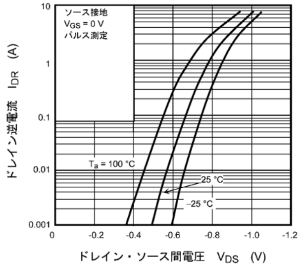
図 7.8 I_{DR} - V_{DS}
