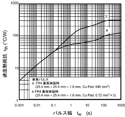
図 7.13 r_{th} - t_w
