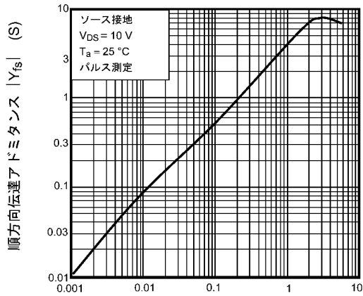
図 8.7 |Y_{fs}| - I_D
