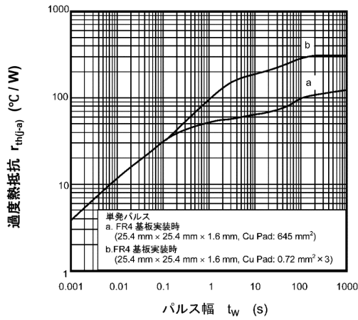
図 8.13 r_{th(j-a)} - t_w
