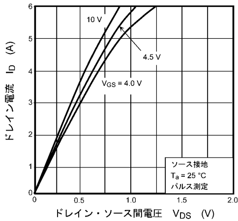
図 7.1 I_D - V_{DS}
