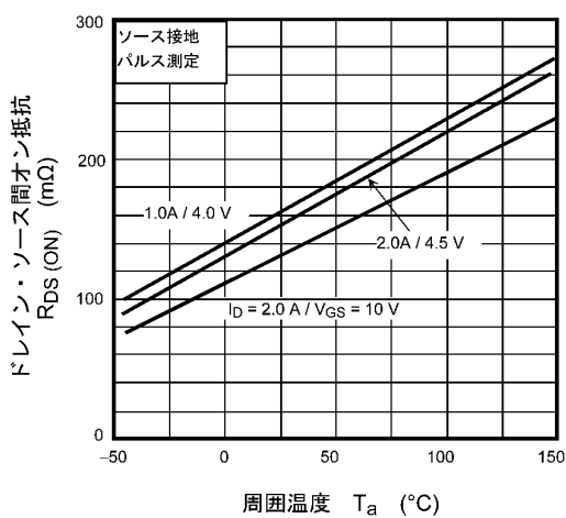
図 8.5 R_{DS(ON)} - T_a
