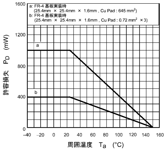
図 7.15 P_D - T_a
