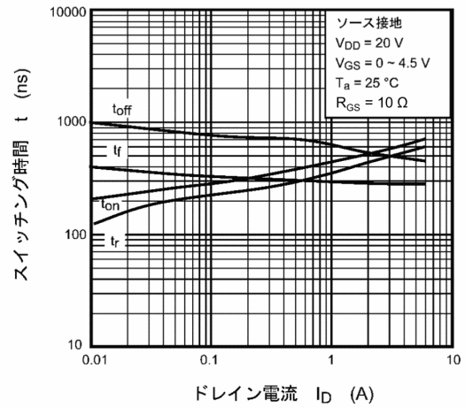
図 8.10 t - I_D
