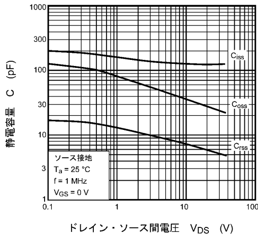
図 8.9 C - V_{DS}
