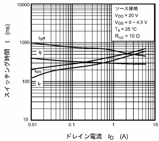
図 7.10 t - I_D
