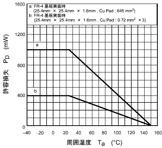
図 8.15 P_D - T_a
