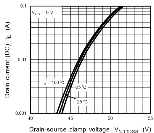
Fig. 7.12 I_D - V_{(CL)DSS}
