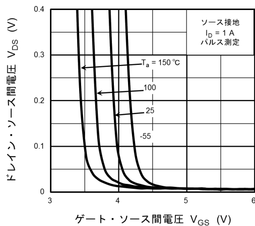
図 8.6 V_{DS} - V_{GS}
