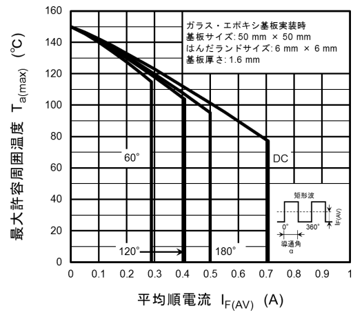
図 10.4 T_{a(max)} - I_{F(AV)}
