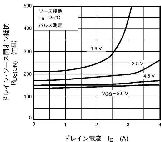
図 7.1.5 R_{DS(ON)} - I_D
