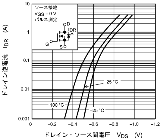
図 7.1.9 I_{DR} - V_{DS}
