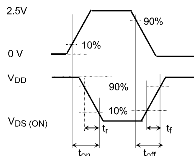
図 5.2.2 入力波形/出力波形
