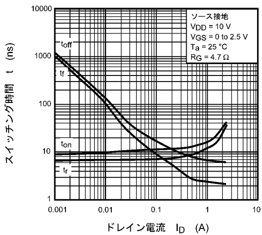
図 7.1.11 t - I_D
