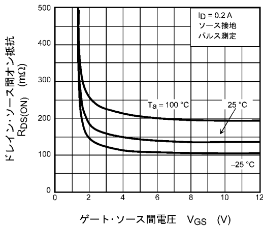
図 7.1.3 R_{DS(ON)} - V_{GS}
