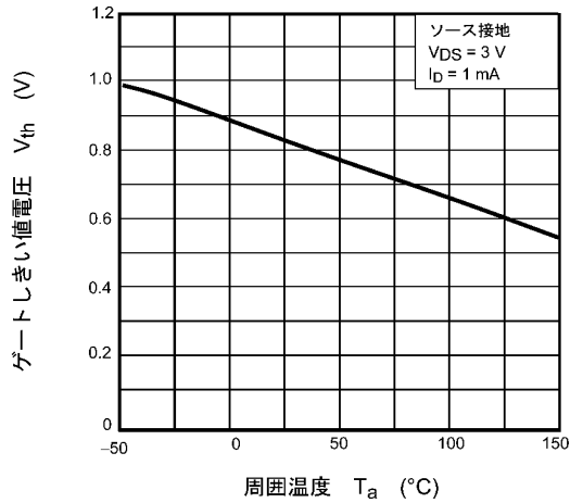
図 7.1.7 V_{th} - T_a
