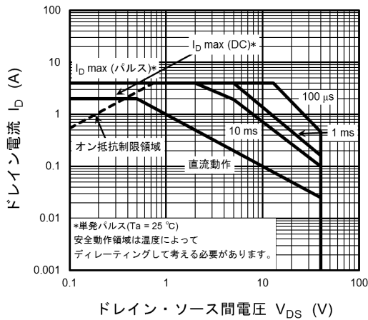
図 7.3.3 安全動作領域
