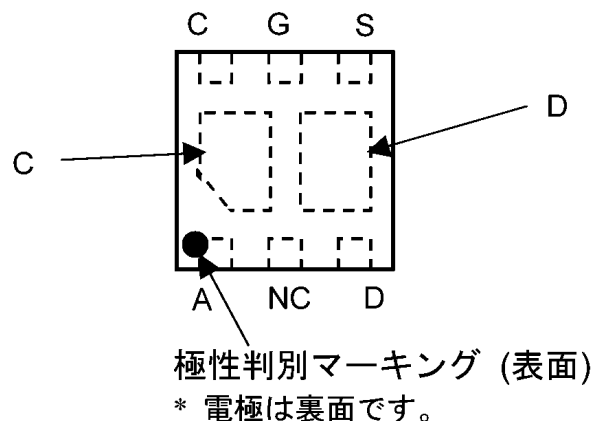
図 6.2 ピン配置(Top View)
