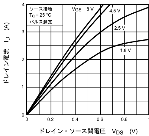
図 7.1.1 I_D - V_{DS}
