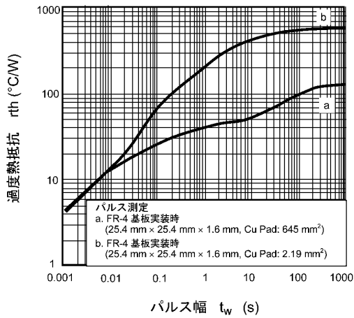
図 7.3.1 r_{th} - t_w
