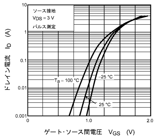
図 7.1.2 I_D - V_{GS}
