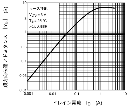
図 7.1.8 |Y_{fs}| - I_D
