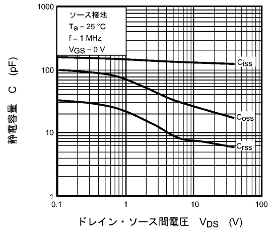
図 7.1.10 C - V_{DS}
