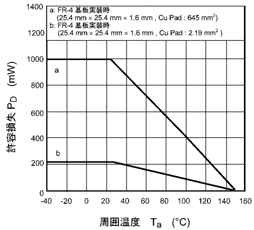
図 7.3.2 P_D - T_a
