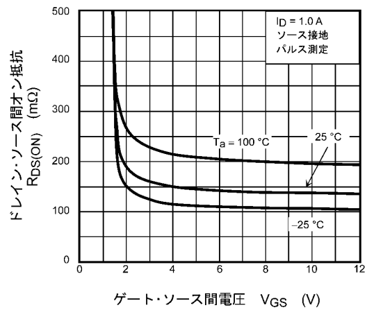
図 7.1.4 R_{DS(ON)} - V_{GS}
