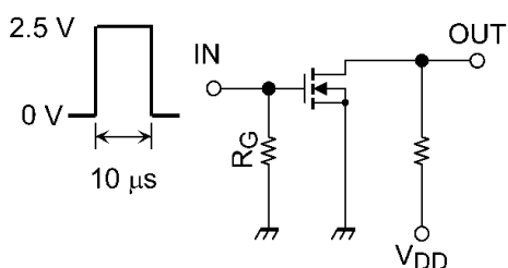
図 5.2.1 スwitching時間の測定回路例
