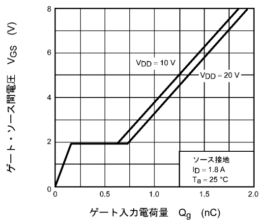
図 7.1.12 ダイナミック入力特性
