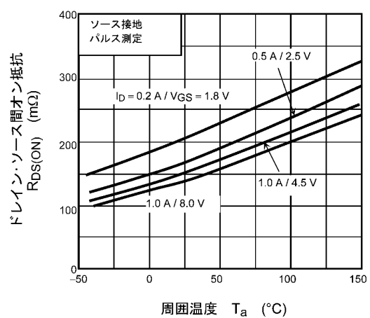
図 7.1.6 R_{DS(ON)} - T_a
