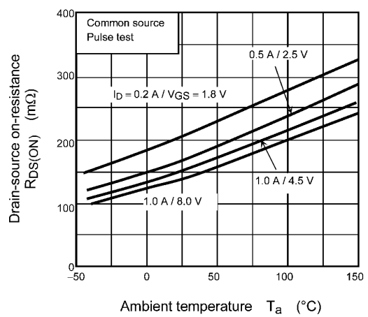
Fig. 7.1.6 R_{DS(ON)} - T_a
