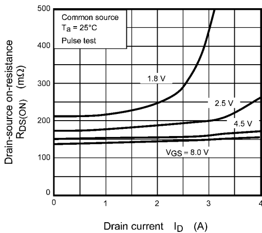
Fig. 7.1.5 R_{DS(ON)} - I_D
