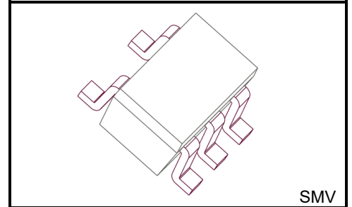
質量: SMV (SOT-25) (SC-74A) : 16 mg (標準)
