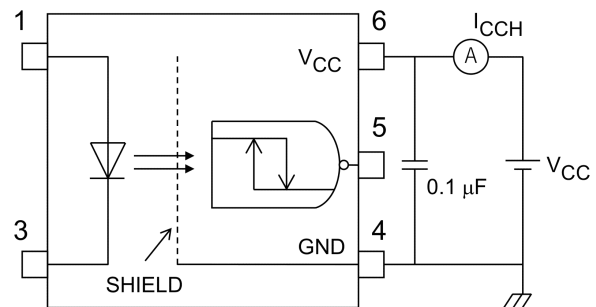
図 12.1.4 I_{CCH} 測定回路
