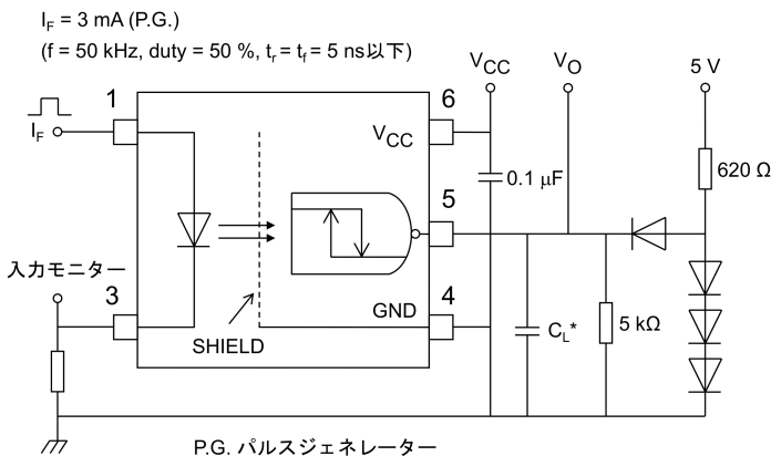
図 12.1.7 伝搬遅延時間測定回路, 波形
