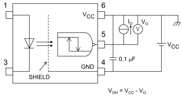
図 12.1.2 V_{OH} 測定回路
