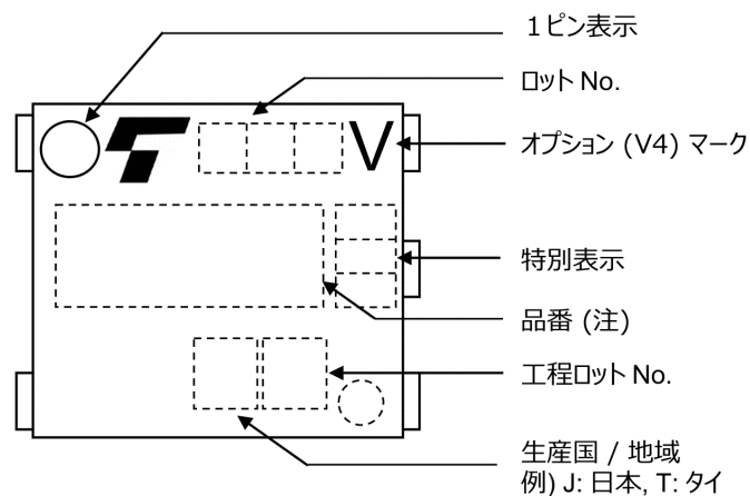
図 16.4 現品表示例 (注)
