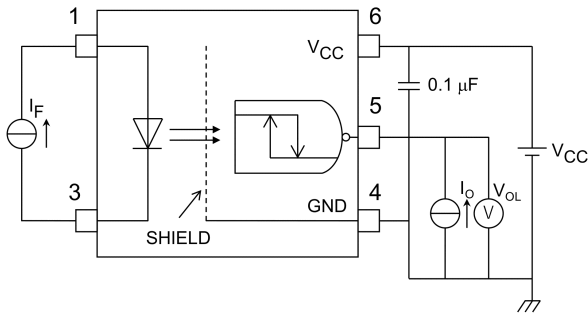
図 12.1.1 V_{OL} 測定回路
