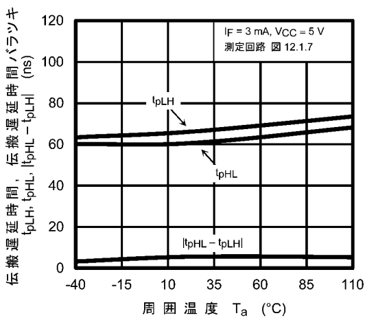
図 12.2.11 t_{pLH} , t_{pHL} , |t_{pHL} - t_{pLH}| - T_a (測定回路 図12.1.7)
