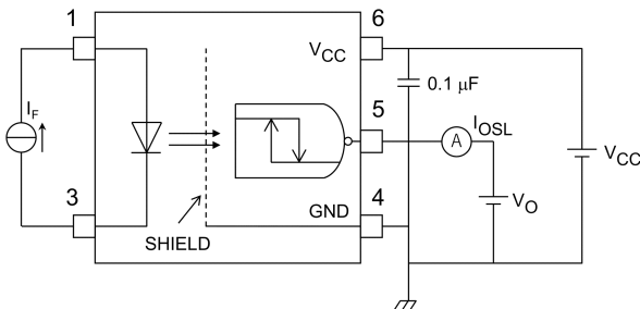
図 12.1.5 I_{OSL} 測定回路
