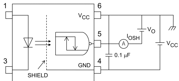
図 12.1.6 I_{OSH} 測定回路
