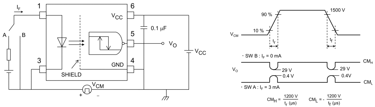
図 12.1.9 コモンモード過渡耐性測定回路, 波形
