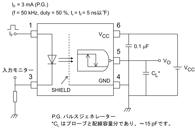
図 12.1.8 伝搬遅延時間測定回路, 波形
