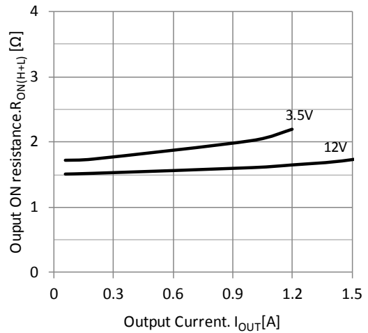
Fig.6 出力オン抵抗( T_a=25^\circ C )
