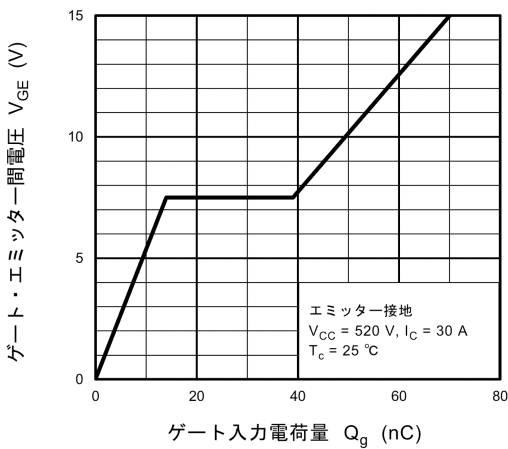
図 8.9 V_{GE} - Q_g
