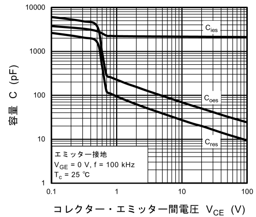
図 8.10 C - V_{CE}
