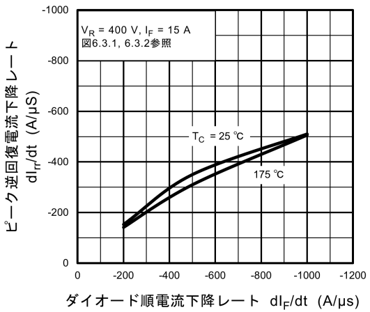
図 8.24 di_{rr}/dt - di_F/dt
