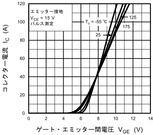
図 8.7 I_C - V_{GE}
